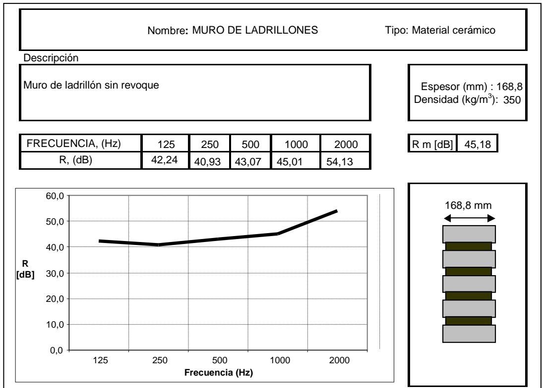
Figura 5: Ficha y gráfico resumen con resistencias acústicas obtenidas sobre muro de ladrillón sin revoque.
